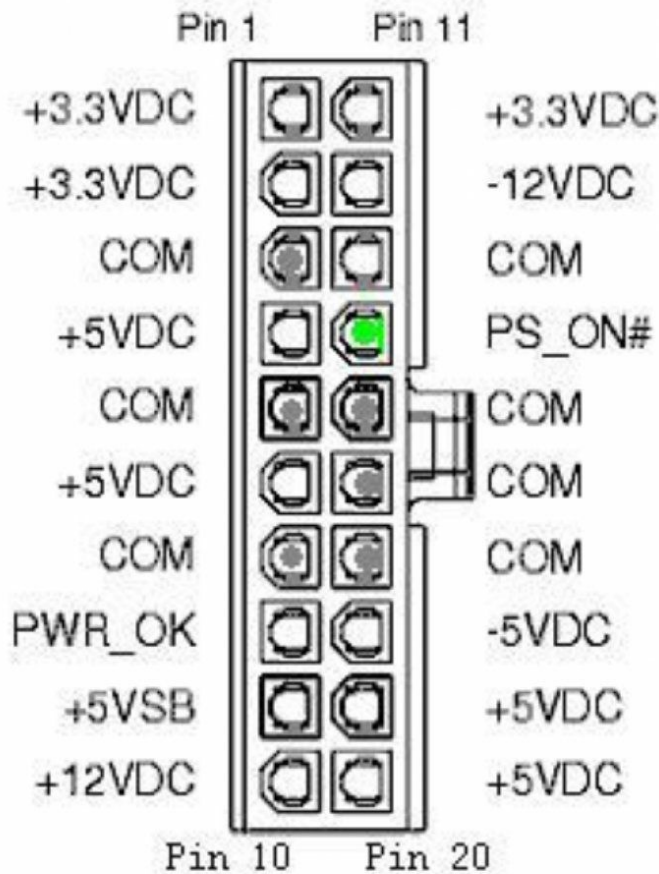
ATX主板电源接口
