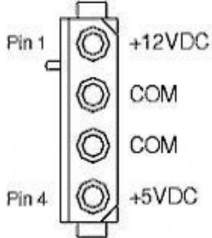
硬盘、光驱电源接口
